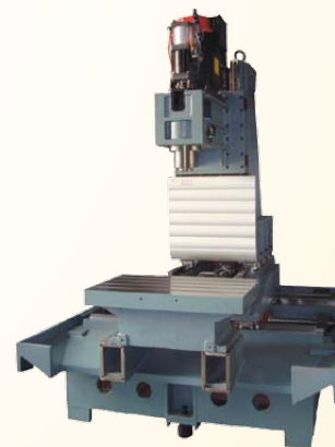
Struttura macchina senza tavola basculante Machine frame without rotary table
